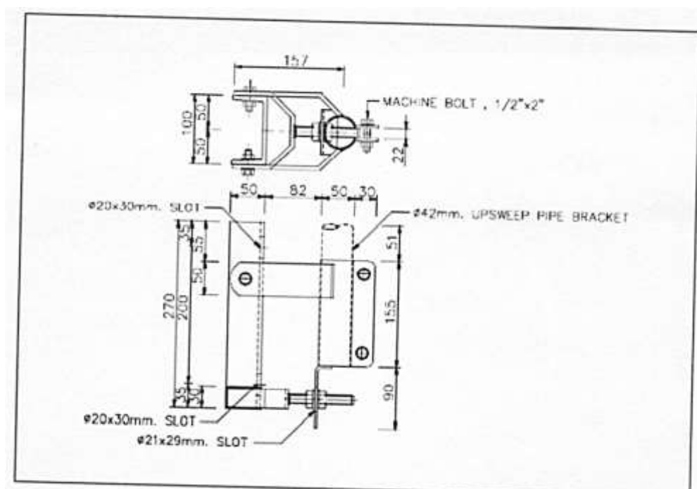
รูปที่ 1-3 กิ่งโคมไฟฟ้า (Rod หรือ Arm) อุปกรณ์ที่เชื่อมต่อกับโคมไฟฟ้า และแป้นติดกิ่งโคมเพื่อยื่นออกไปให้แสงสว่างแก่บริเวณที่ต้องการ
